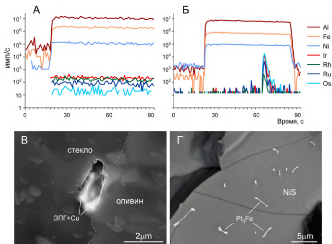
Рисунок 20. Формы выделения ЭПГ в магматических и мантийных породах. (А, Б) разрешенные во времени спектры лазерной абляции. (А) гомогенная окисленная хромшпинель, гарцбургиты Шивелуча. (Б) включение осмистого иридия в магматической Cr-шпинели, Толбачик. (В) Включения металлического сплава в базальтовом стекле, влк. Толбачик: \text{Cu} \approx \text{Ir} > \text{Rh} > \text{Pd} > \text{Pt} > \text{Os} > \text{Ru} ; \Sigma \text{ЭПГ} \approx 75 \text{ мас.}\% . (Г) Исоферроплатина ( \text{Pt}_3\text{Fe} ) на поверхности сульфида ( \text{NiS} ), гарцбургиты, влк. Шивелуч.
