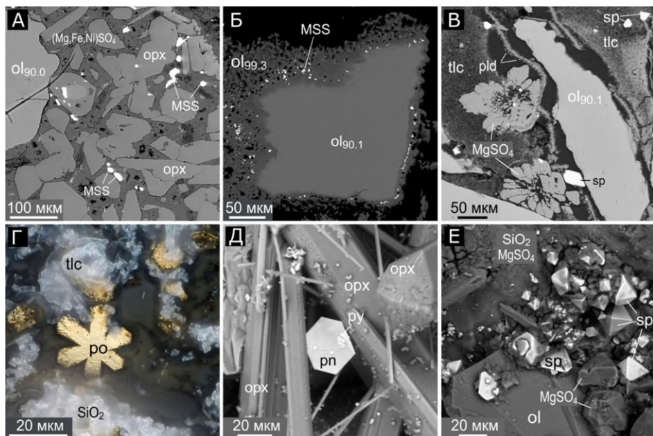
Рисунок 6. Экспериментальные продукты при 0,5 ГПа и 1000 °C. (А) Безводная система оливин– \text{SO}_2 : исходный оливин окружен ортопироксеном и глобулами MSS в сульфатной матрице (\text{Mg,Fe,Ni})\text{SO}_4 . (Б–Е) Система оливин– \text{H}_2\text{O} – \text{SO}_2 : (Б) Оливин ( \text{Mg\# } 90,1 ), частично замещен высокомагнезиальным оливином ( \text{Mg\# } 93,0\text{--}99,3 ), с глобулами MSS в межзерновых пустотах. (В) Фрагменты исходного оливина в матрице из безводного \text{MgSO}_4 и волокнистого талька. (Г) Гексагональный циклический двойник пирротина, окруженный тальком и аморфным кремнеземом \text{SiO}_2 \cdot n\text{H}_2\text{O} . (Д) Игольчатый и призматический ортопироксен, гексагональный пентландит ( \text{Ni}_{4.1}\text{Fe}_{4.9}\text{S}_8 ), на поверхности кристаллов мелкий закалочный пирит. (Е) Шпинель и \text{MgSO}_4 на поверхности оливина. Методы: (Г) – оптическая микроскопия; остальные – электронные микрофотографии (отраженные электроны). Редокс-условия: (А) – без буфера; (Б) – внешний буфер IW; (Б–Д) – без буфера ( \sim \text{NNO} ); (Е) – внешний буфер МН. Сокращения: ol – оливин; opx – ортопироксен; pn – пентландит; po – пирротин; py – пирит; sp – шпинель; tlc – тальк.
