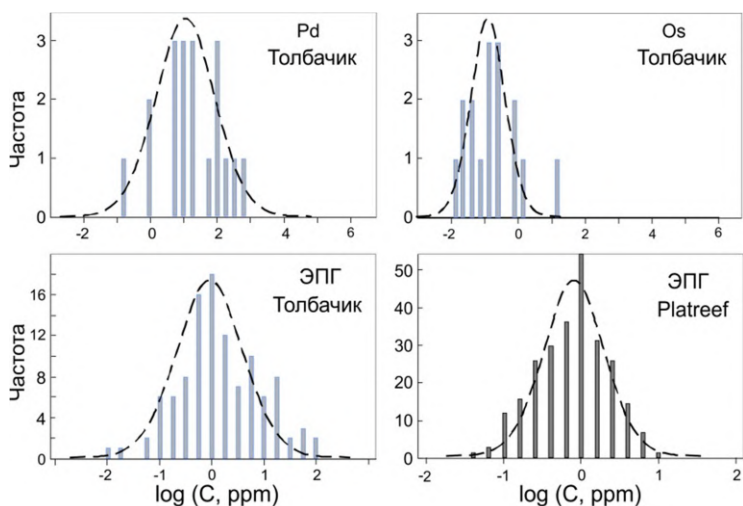
Рисунок 17. Гистограммы частот для логарифмов концентраций Pd, Os и суммы ЭПГ в сульфиды Толбачика. Для сравнения показана распределение для сульфидов Платриф, Южная Африка. Гистограммы для логарифмов концентраций ЭПГ близки к теоретической линии нормального распределения (пунктир).
