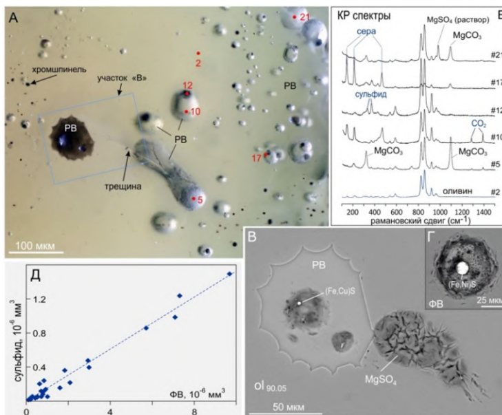
Рисунок 5. Флюидные включения (ФВ) в оливине. (А) Кристалл оливина с роем многофазных ФВ, а также расплавленное включение. Прямоугольником отмечена область, показанная на (В); пронумерованные метки показывают места отбора спектров КР. (Б) КР (Рамановские) спектры ФВ. (В) Область «В», видны расплавленное включение (РВ) и высохшая флюидная капля ( \text{MgSO}_4 ) после декрепитации флюидного включения. Контракционный пузырь РВ содержит каплю Fe-Cu сульфида. (Г) Вскрытое ФВ с глобулой Fe-Ni сульфида. (Д) Объемы сульфидных глобул внутри ФВ коррелируют с объемами ФВ в пределах двух порядков величины.
