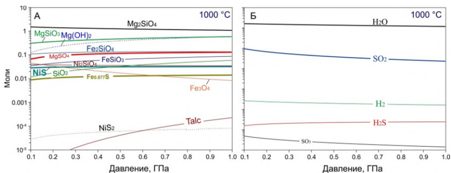
Рисунок 8. Равновесные фазовые составы в системе оливин-Н 2 О-SO 2 , при постоянной температуре 1000 °С и давлениях 0,1–1,0 ГПа.
