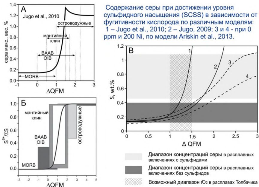
Рисунок 14. Содержание серы в расплаве (А), доля сульфатной серы (Б) и содержание общей серы в расплаве при достижении сульфидного насыщения (В) в зависимости от фугитивности кислорода, выраженной в логарифмических единицах в виде \Delta QFM .
