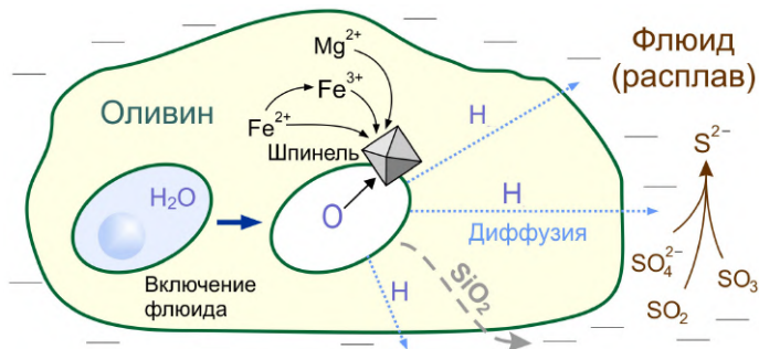
Рисунок 4. Схема взаимодействия оливина и флюидного включения с водой. Вода окисляет \text{Fe}^{2+} в оливине; окисленное железо \text{Fe}^{3+} консервируется в кристалле шпинелида – магнезиального магнетита (обычно, одиночном). Условиями диффузионного оттока водорода из зоны реакции является разность химических потенциалов ( \mu_{\text{H}_2} ) внутри включения и снаружи кристалла.
