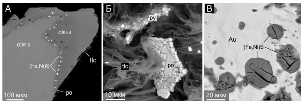
Рисунок 7. Экспериментальные продукты при 2,8 ГПа и 1000 °С, система оливин– H_2O – SO_2 . (А) Частичное замещение оливина (Mg# 89,0) более магнезиальной фазой (Mg# 95,4), глобулы MSS занимают пустоты между высоко- и низкомагнезиальным оливином. (Б) Гексагональные кристаллы пирротина, обросшие мелкими кристаллами закалочного пирита; листоватый тальк на заднем плане. (В) Глобулы MSS, содержащие 6-8 мас.% Ni на внутренней поверхности золотой ампулы. Сокращения минералов соответствуют Рис. 6.
