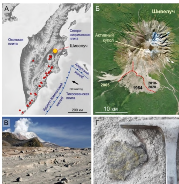
Рисунок 9. Вулкан Шивелуч и объекты исследования. (А) Расположение вулкана Шивелуч и других действующих вулканов Камчатки. (Б) Спутниковый снимок Шивелуча, показывающий недавние пирокластические потоки, по состоянию на июль 2022 года. Цифрами обозначены отложения обломочной лавины 1964 года и пирокластических потоков 2005 и 2010-2020 годов. (В) Пирокластический поток извержения 2005 года протяженностью 18 км состоит из несортированного
